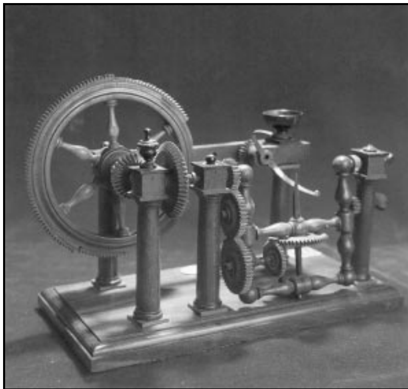
Fig.- Modelo de máquina devanadora. Museo Central del Transporte Ferroviario, San Petesburgo. KP, 1913
